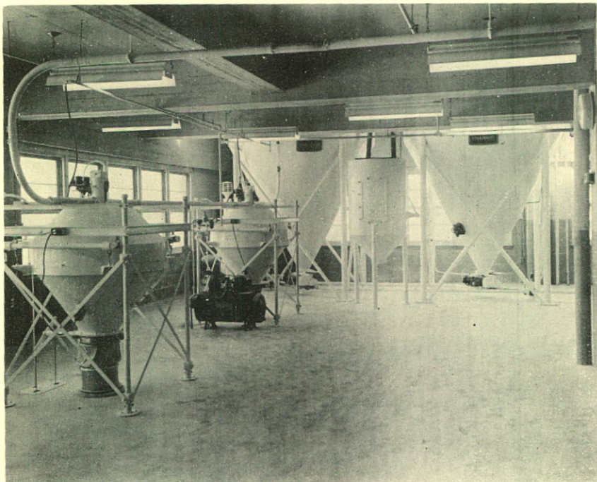
RÉSERVOIRS ET BALANCES AUTOMATIQUES POUR FARINE.
