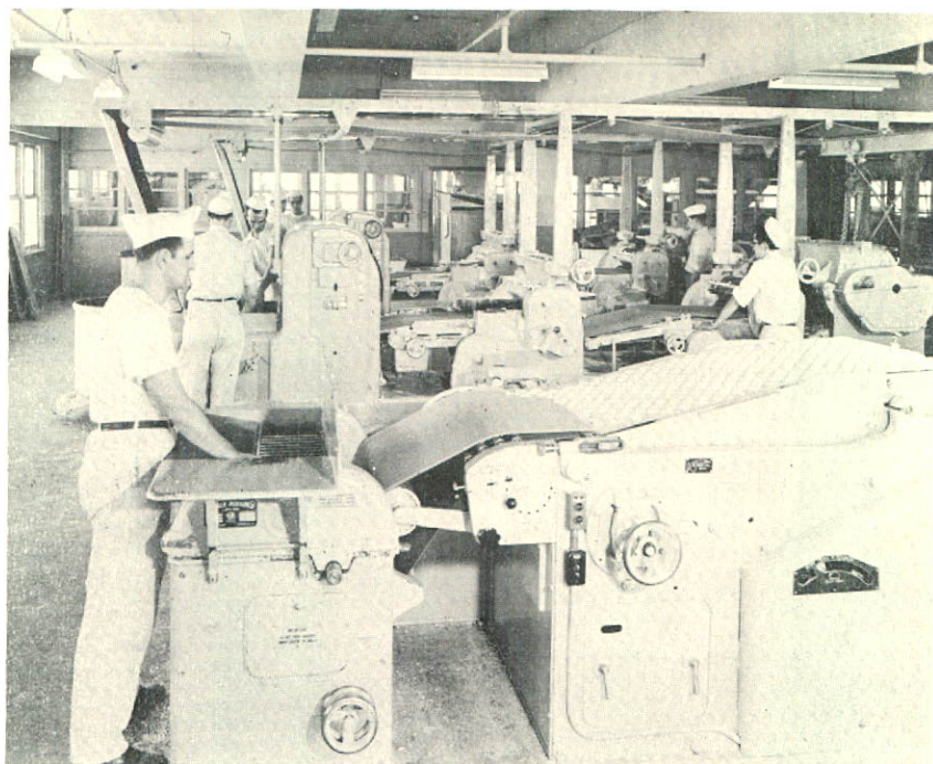
MOULEUSE ET DÉCOUPEUSES A BISCUITS.
