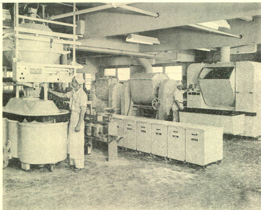
SECTION DE LA PRÉPARATION DES PÂTES: PESÉE AUTOMATIQUE DE LA FARINE ET MALAXEURS À PÂTE.
