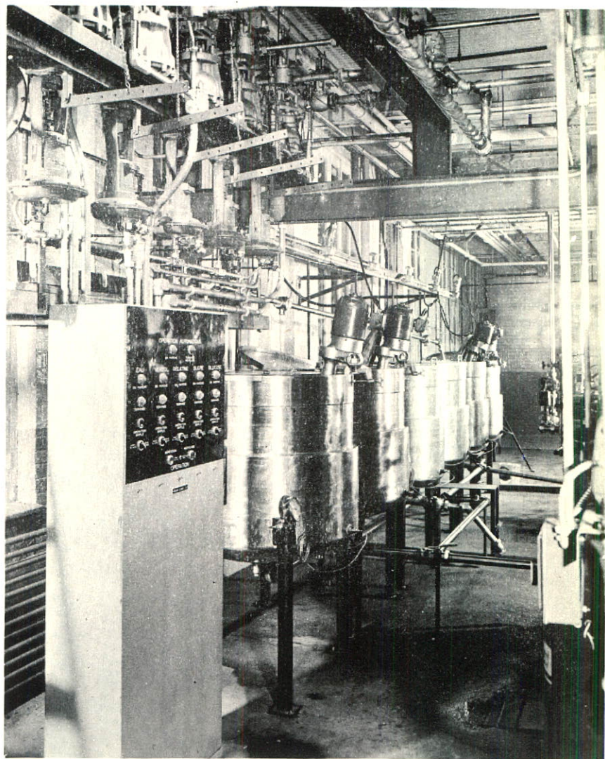
PANNEAU DE CONTRÔLE ET SÉRIE DE BASSINS POUR LA PRÉPARATION AUTOMATIQUE DE LA GUIMAUVE.
