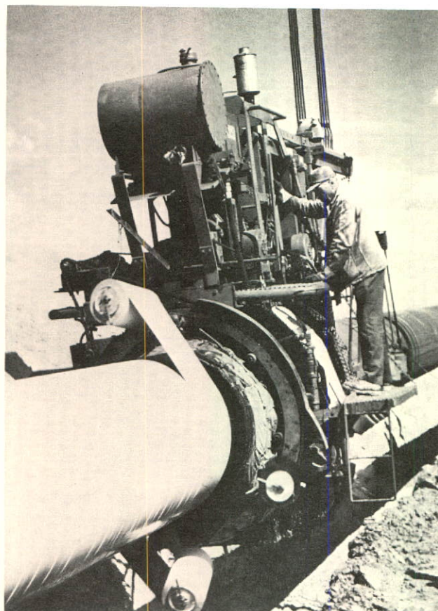
Enrobage du pipe-line à l'endroit où il traversera la Saskatchewan-Sud dans l'est de l'Alberta.
