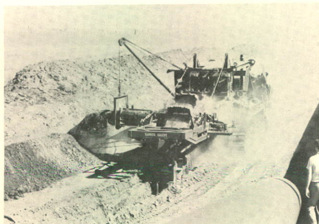
Creusage dans les Grandes collines Sand de la Saskatchewan. Cette trancheuse peut creuser un fossé de 3m (10 pi) de profondeur et de 2m (6,5 pi) de largeur de sorte qu'un minimum de 0,8m (3 pi) de terre recouvre le pipe-line.
