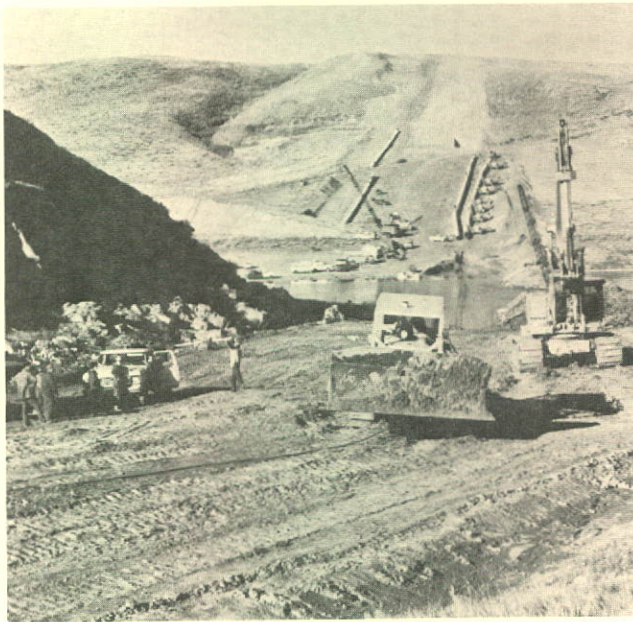
Le pipe-line traverse la Saskatchewan-Sud, dans l'est de l'Alberta. Alors qu'une grue latérale submerge le premier tronçon, un boteur, ancré sur la rive opposée, le hale à l'aide de câbles.
