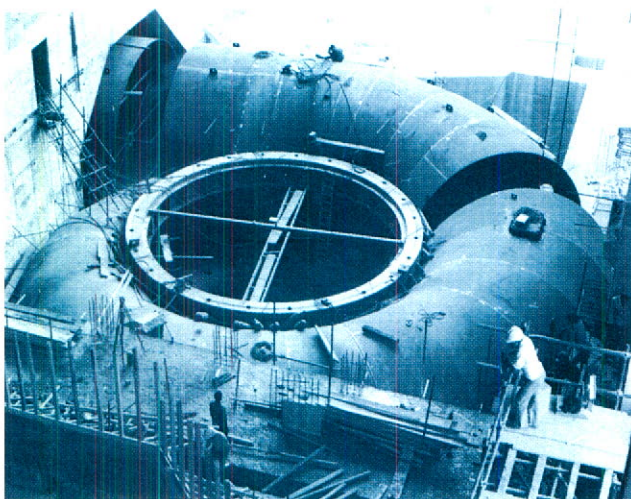
CENTRALE ELECTRIQUE AU NIGERIA – L'expansion de cette centrale électrique à Kainji, complétée l'an dernier, nous a valu un prix de l'Association des ingénieurs-conseils du Canada. Les ingénieurs de Monenco ont conçu de nouvelles unités pouvant produire 60 pour cent plus d'énergie à même l'espace déjà existant dans la centrale.
